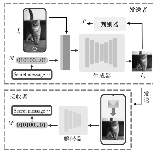
图 1 基于 GAN 的移动端隐写方法整体结构
