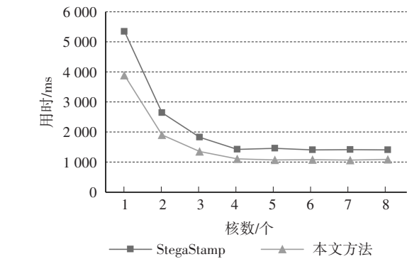
图 4 不同 CPU 核数下运行模型所需时间
