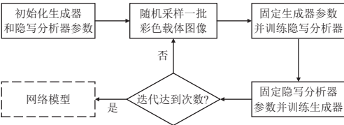
图 4 CIS-GAN 整体训练流程框图
